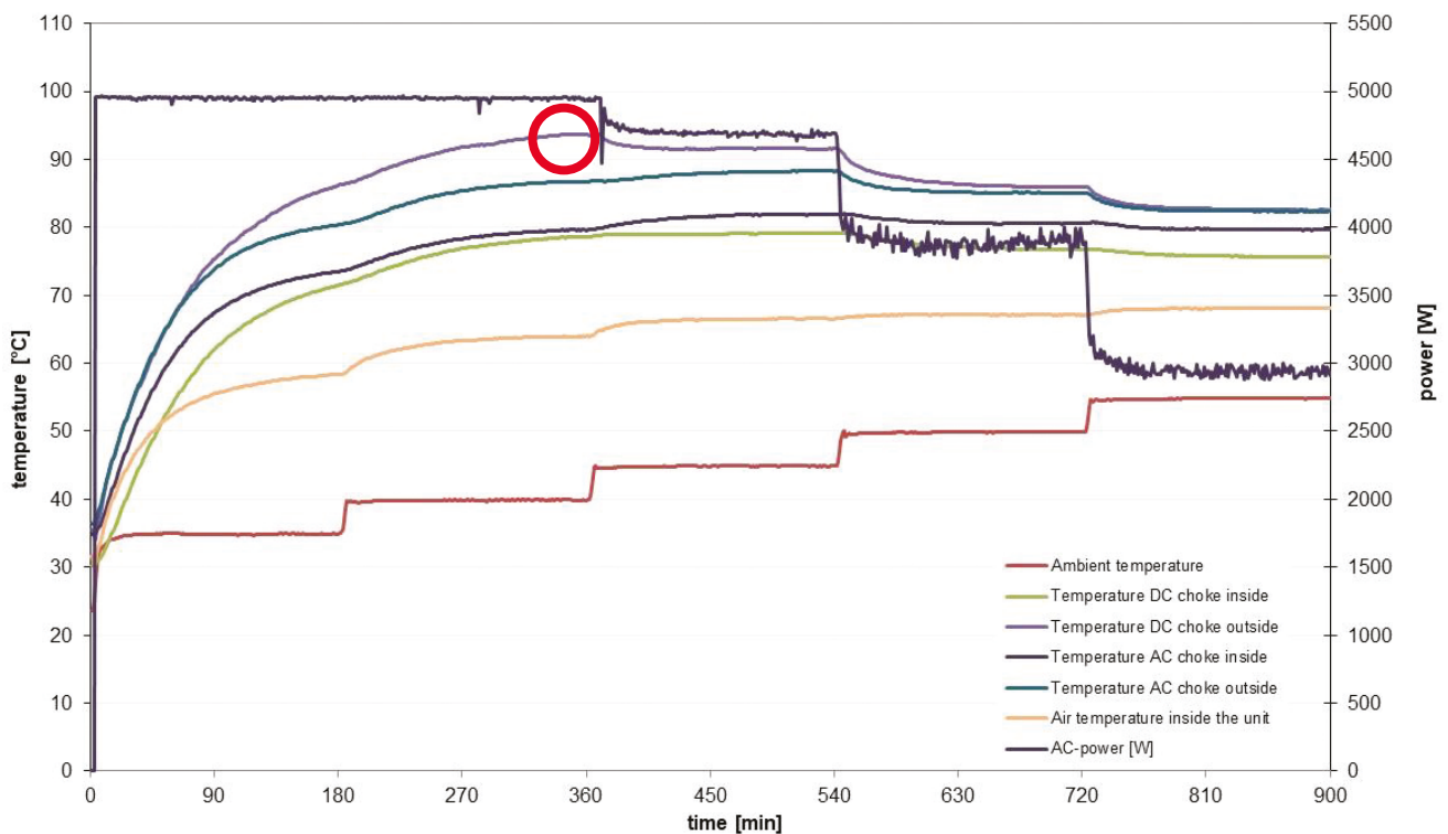
Rysunek 15: Wykres temperatury otoczenia i mocy wyjściowej dla aktywnie chłodzonego falownika Fronius
