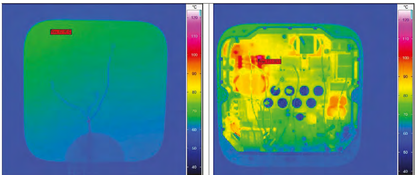
Rysunek 12: Dystrybucja ciepła w pasywnie chłodzonym falowniku w temperaturze otoczenia 55 °C ( P_{AC} = 5 kW, U_{mpp} = 260 V) [źródło: Fronius]
