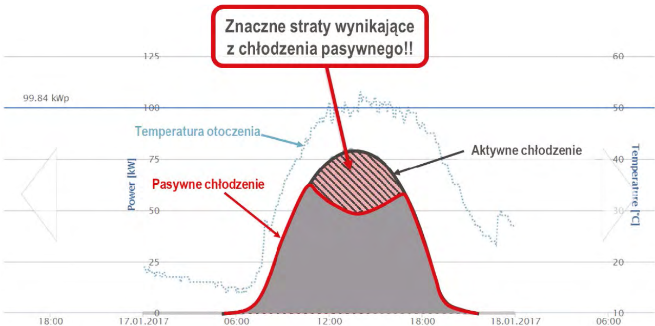
Rysunek 11: Należy oczekiwać spadku wydajności lub straty przy chłodzeniu pasywnym
