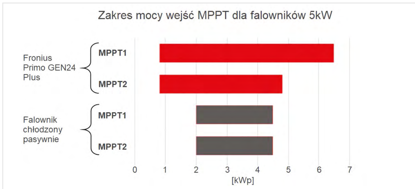
Rysunek 1: Porównanie rozkładu mocy trackera MPP dla pasywnie i aktywnie chłodzonych falowników 5 kW
