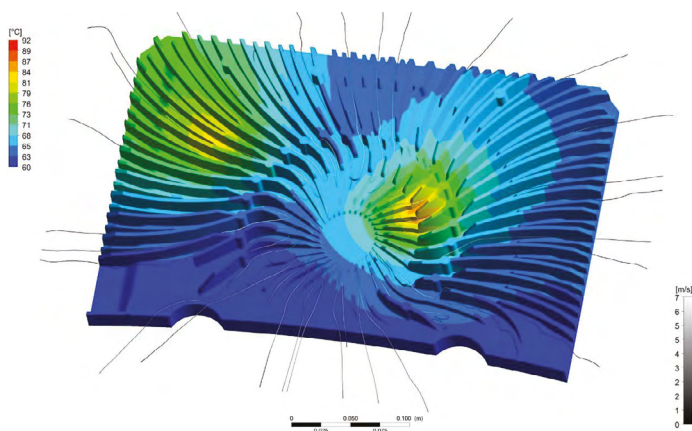
Rysunek 17: Symulacja przepływu CFD - szybkie usuwanie ciepła za pomocą żeber chłodzących radiatora [źródło: Fronius]
