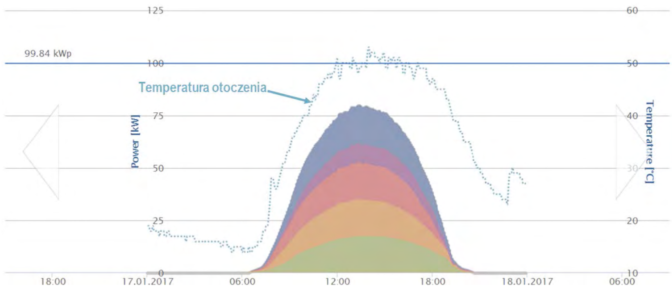
Rysunek 9: Dzienna krzywa wydajności i wykres temperatury otoczenia
