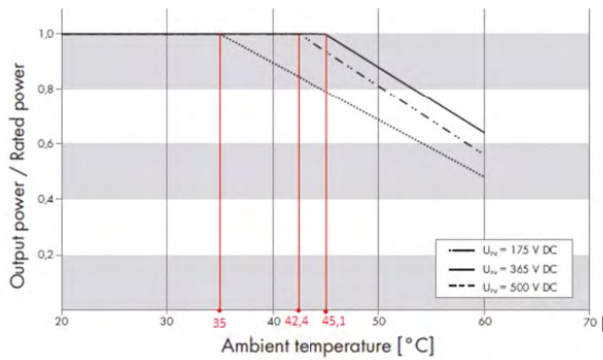
Rysunek 14: Obniżenie mocy zależne od temperatury otoczenia przy P_{AC,nom} = 5 \text{ kW} [źródło: karta danych technicznych firmy konkurencyjnej]
