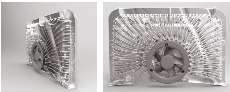
Rysunek 16: Innowacyjny system chłodzenia Fronius GEN24 Plus oraz GEN24 [źródło: Fronius]
